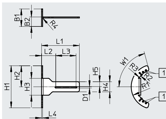
[1] Löcher für Schrauben M4x10
