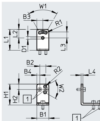
[1] Schraube M4x10
