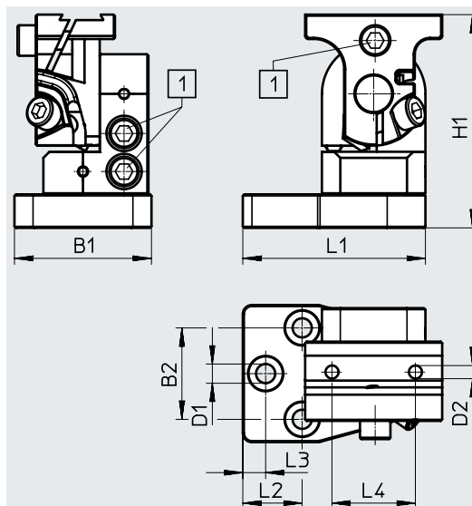
[1] 4x Schraube DIN 912 M6
